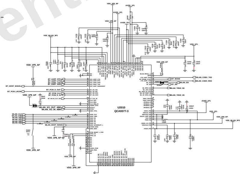
BT/WiFi
